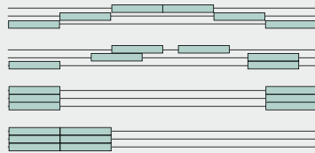
A. Schuifdeur met vrij verplaatsbare vleugels
